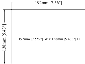
Cutout Dimensions
