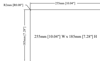
Cutout Dimensions
