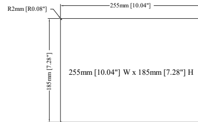
Cutout Dimensions
